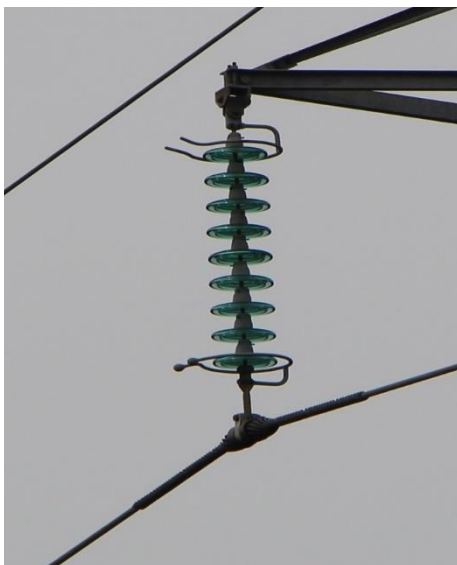
Figur 5. Detalj på isolator som i detta fall hänger nedåt från regeln och utgörs av glasskivor, keramiska skivor eller något gummimaterial. Längden är ofta flera meter på ledningar med högre spänningar. Ju högre spänning desto längre isolator. På stolptyper med stående isolator kan höjden variera mellan ca 20–80 cm.
