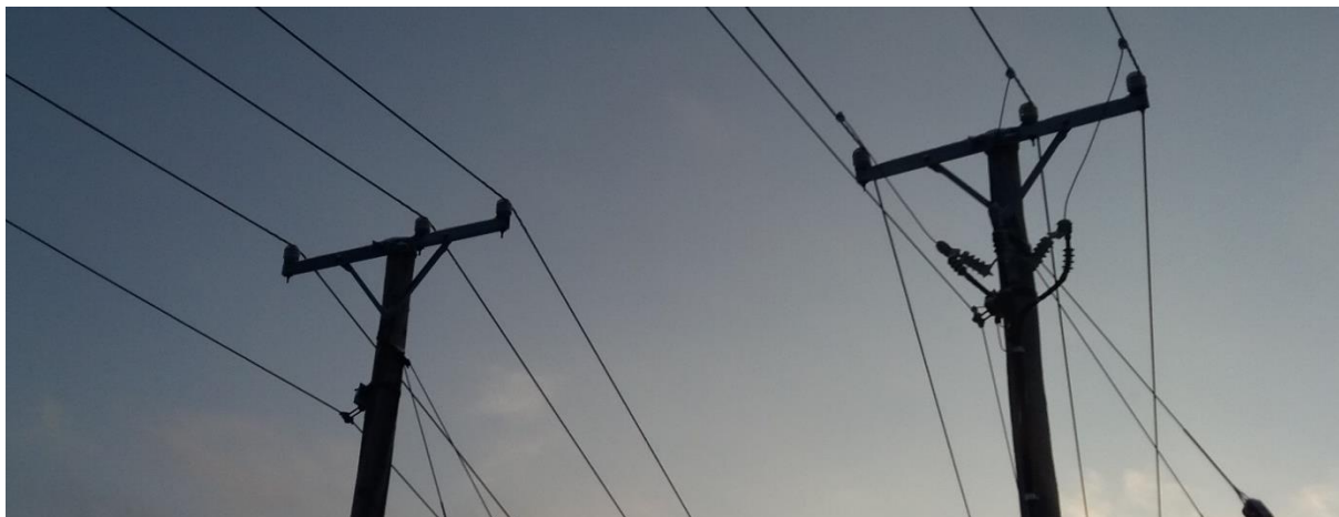
Figur 12. Samma typ av lokalnätsstolpe som i figur 11 med stående isolatorer. Här kan dock ses att faslinorna sitter asymmetriskt, dvs. att två faslinor sitter närmare varandra vilket ger ett kortare avstånd mellan strömförande delar. Konstruktionen är av äldre typ. Till vänster syns en lina under faslinorna, en s.k. längsgående jordlina. I utländska studier benämns den ofta neutralledare.
